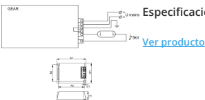
Especificaciones Philips HID-PV C 35 /S CDM 220-240V 50/60Hz
